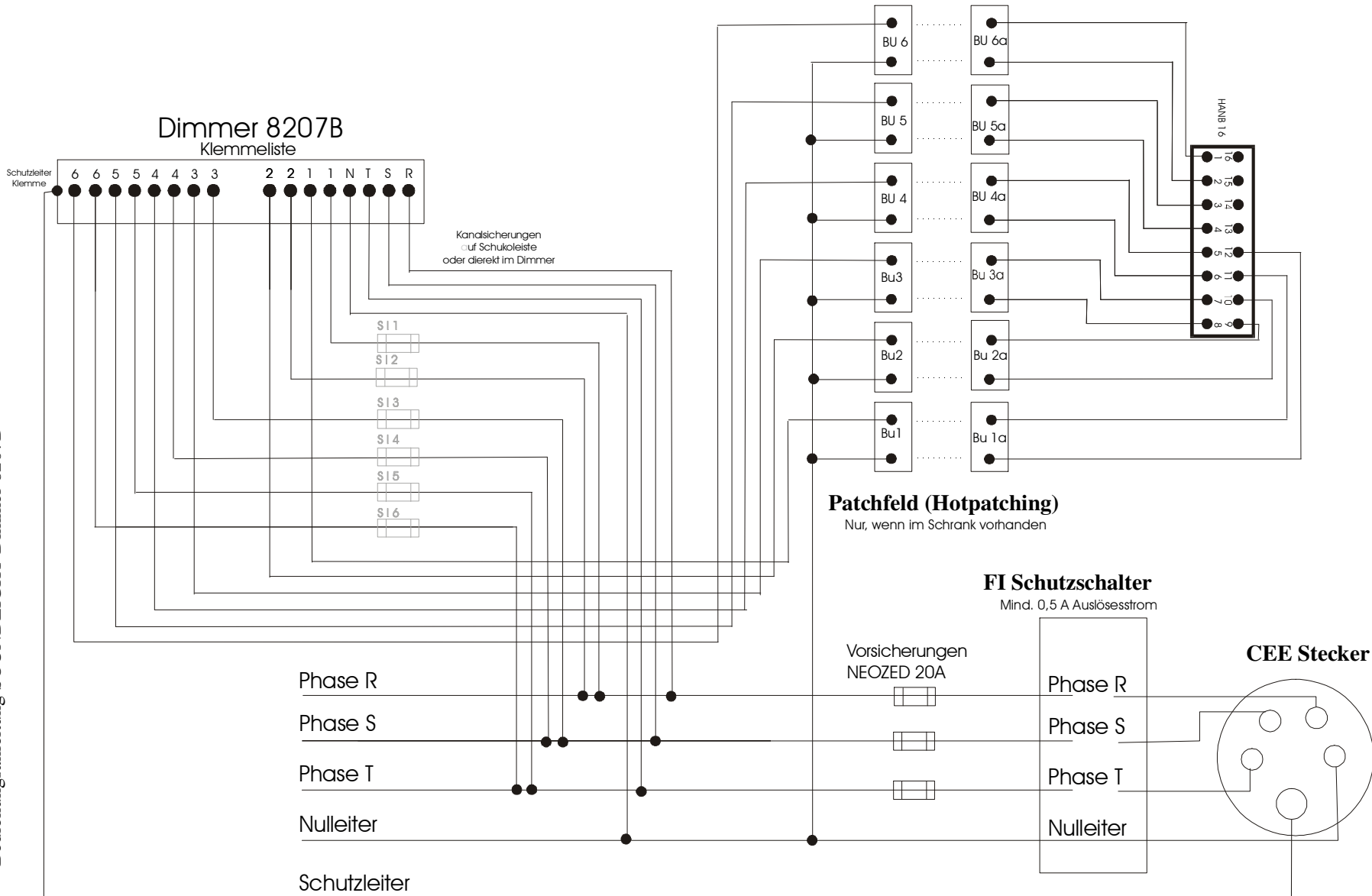
Mindestkonfiguration Anschluss DimmerPack 8207B innerhalb eines Schaltschranks oder Stromverteilung
